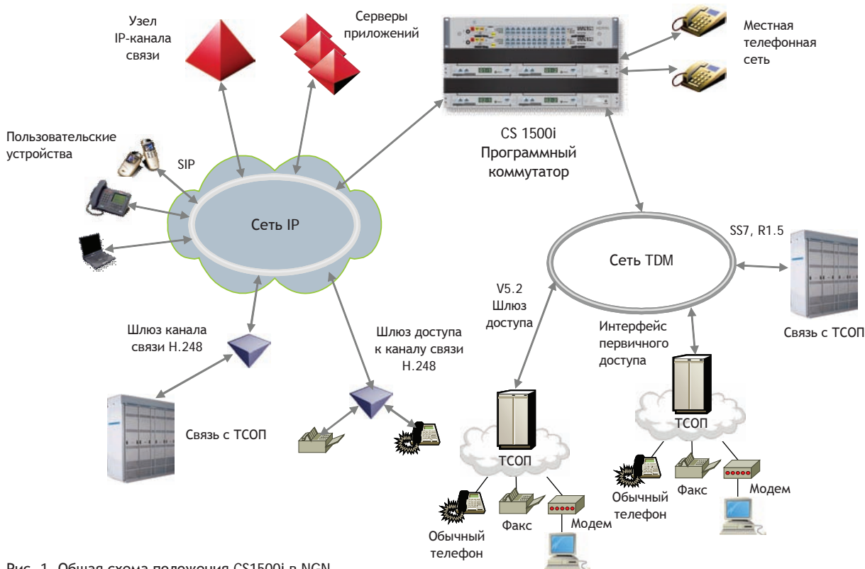
Рис. 1. Общая схема положения CS1500i в NGN
